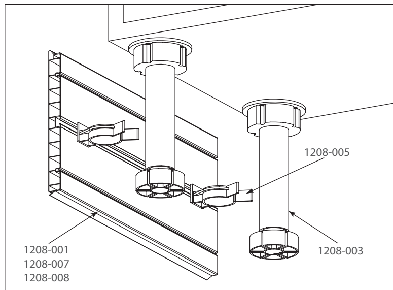
Diagrama de instalación:
