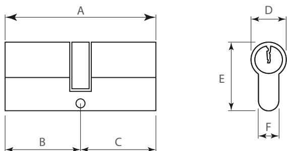
Cilindro llave / llave
