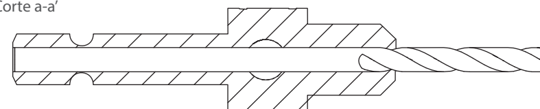
Corte a-a'
