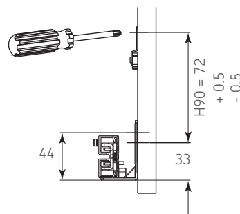
Ensamble Accesorios
