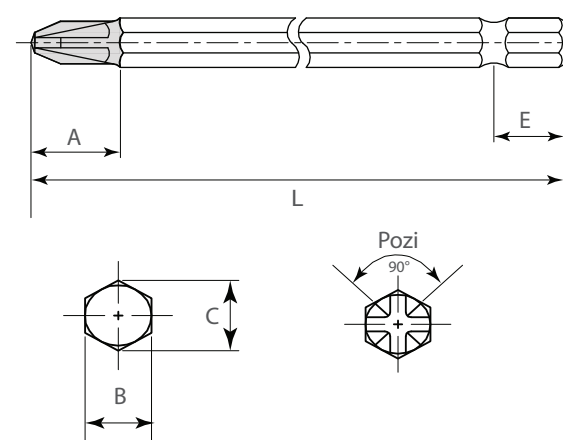
Dimensiones generales
