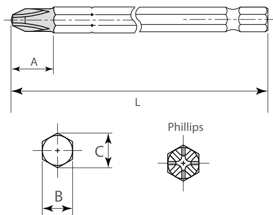
Dimensiones generales
