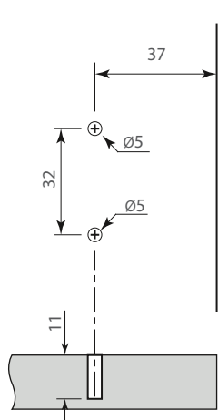
Perforación del gabinete (base)
