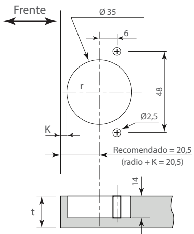
Perforación de la puerta (puerta)
