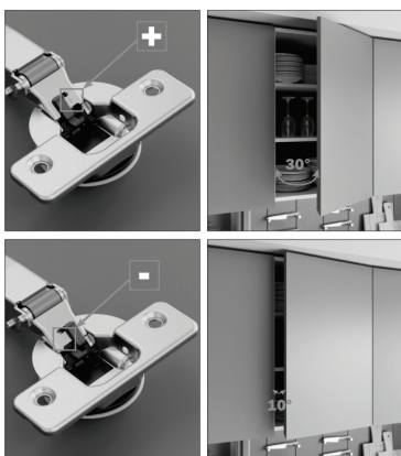
Regulación de la velocidad del cierre suave
