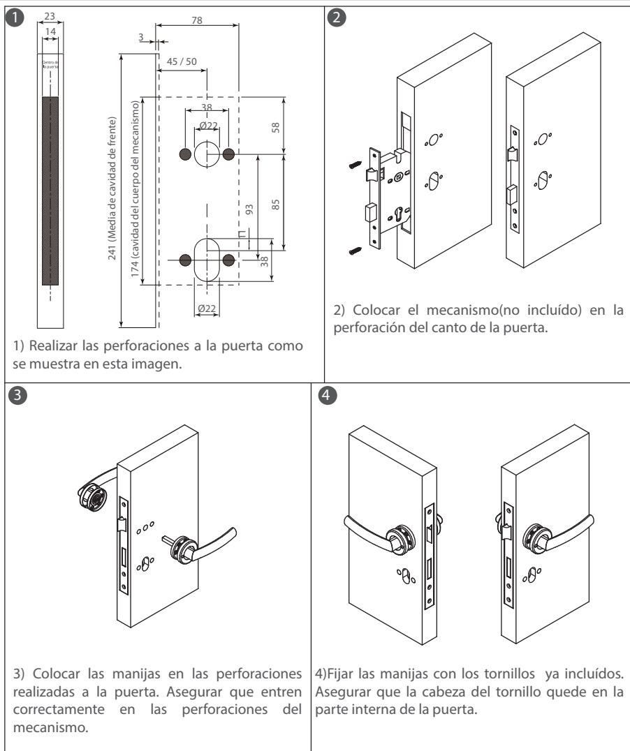
Diagrama de ensamble
