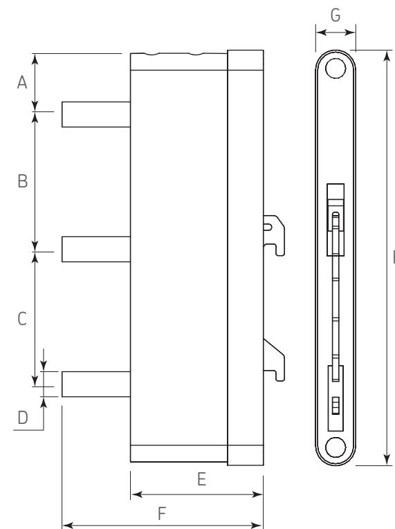
Dimensiones generales
