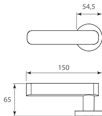
Manija interior
