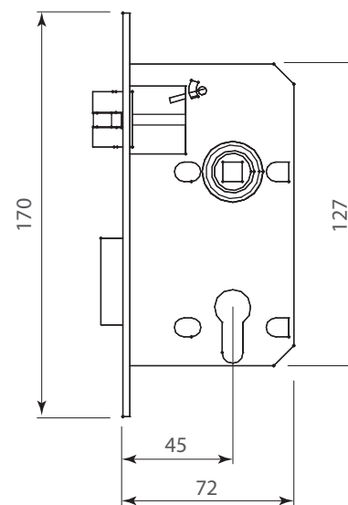
Mecanismo (reversible)
