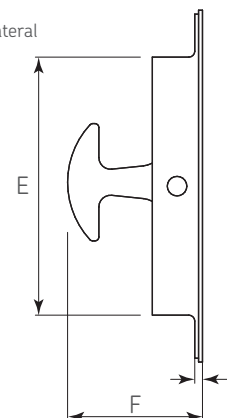
Dimensiones generales
