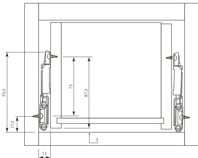
Diagrama de instalación:
