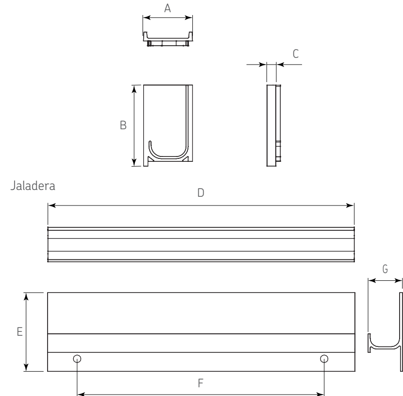
Dimensiones generales
