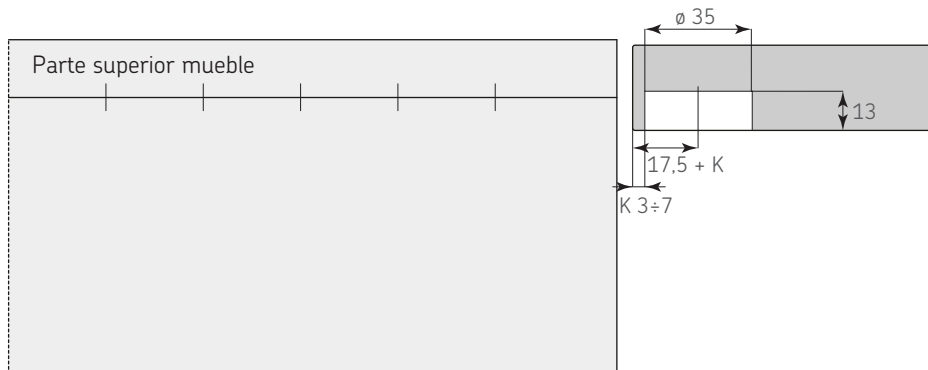
Vista lateral
