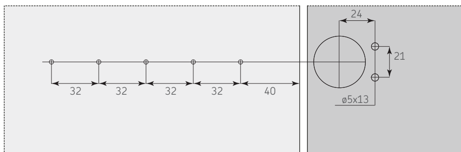
Vista superior
