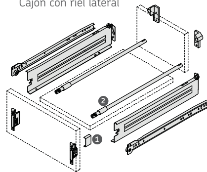
Cajón con riel lateral
