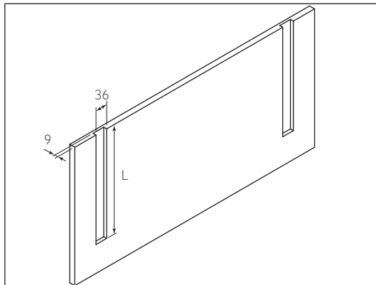
1) Realizar un saque a la puerta de 36 x 9 x L
