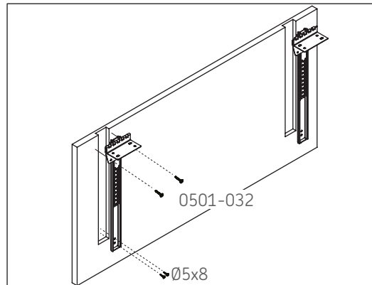
2) Colocar pegamento y fijar las correderas con los tornillos Ø5x8 para la corredera y 0501-032 para el soporte (tornillos no incluidos)
