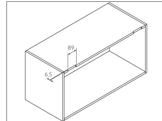
3) Realizar un saque de 6,5 x 89 al techo del gabinete.
