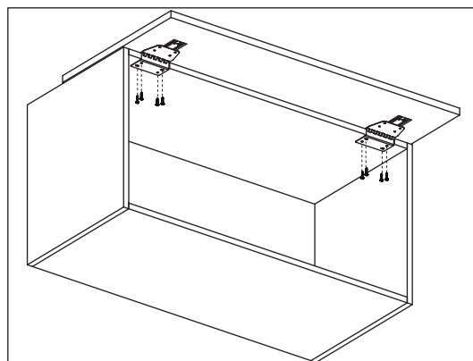
4) Fijar la puerta al techo del gabinete con los tornillos 0501-032 (no incluidos)
