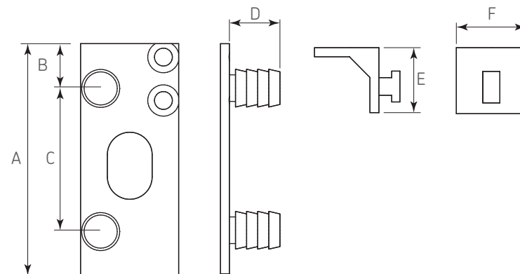
Dimensiones generales
