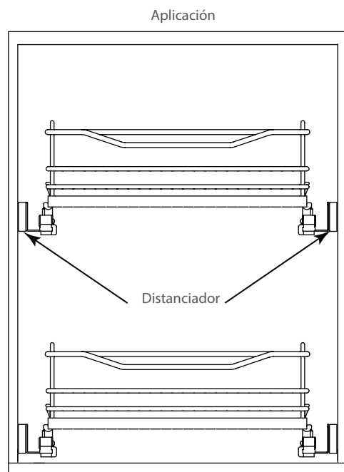
Diagrama de instalación:
