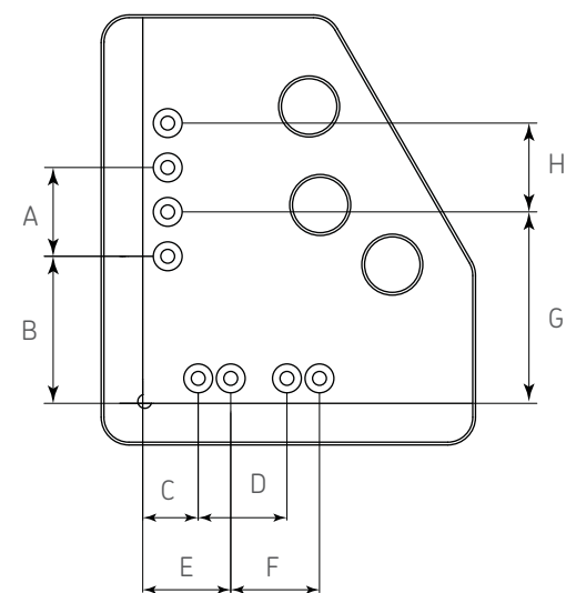
Dimensiones generales
