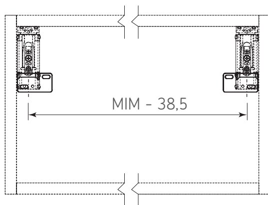
A) Aplicacion para un solo gabinete
