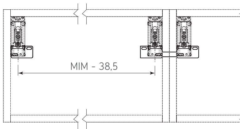
B) Aplicacion para un gabinete junto a otro
