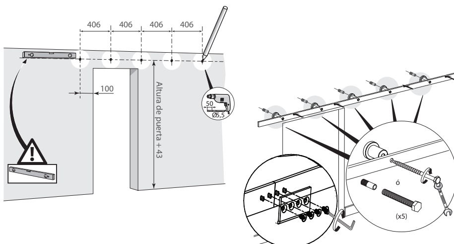
Fijación del conector para el código 0808-010
