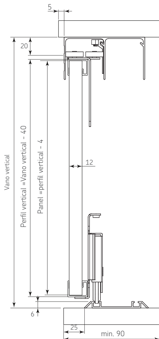
Diagrama de instalación:
