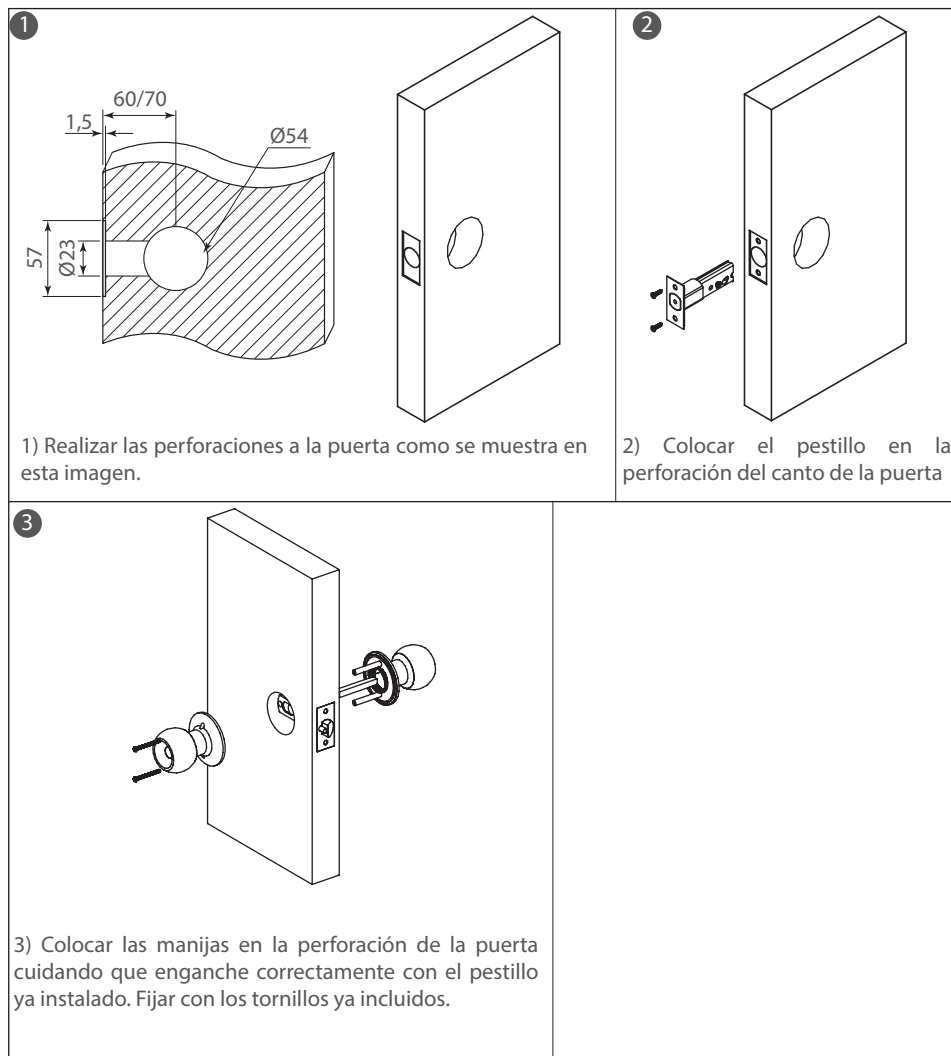
Diagrama de ensamble manija de bola
