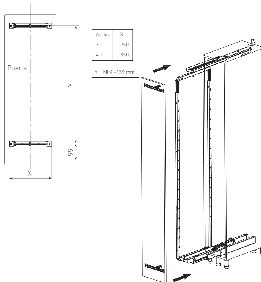
Ensamble de la puerta
