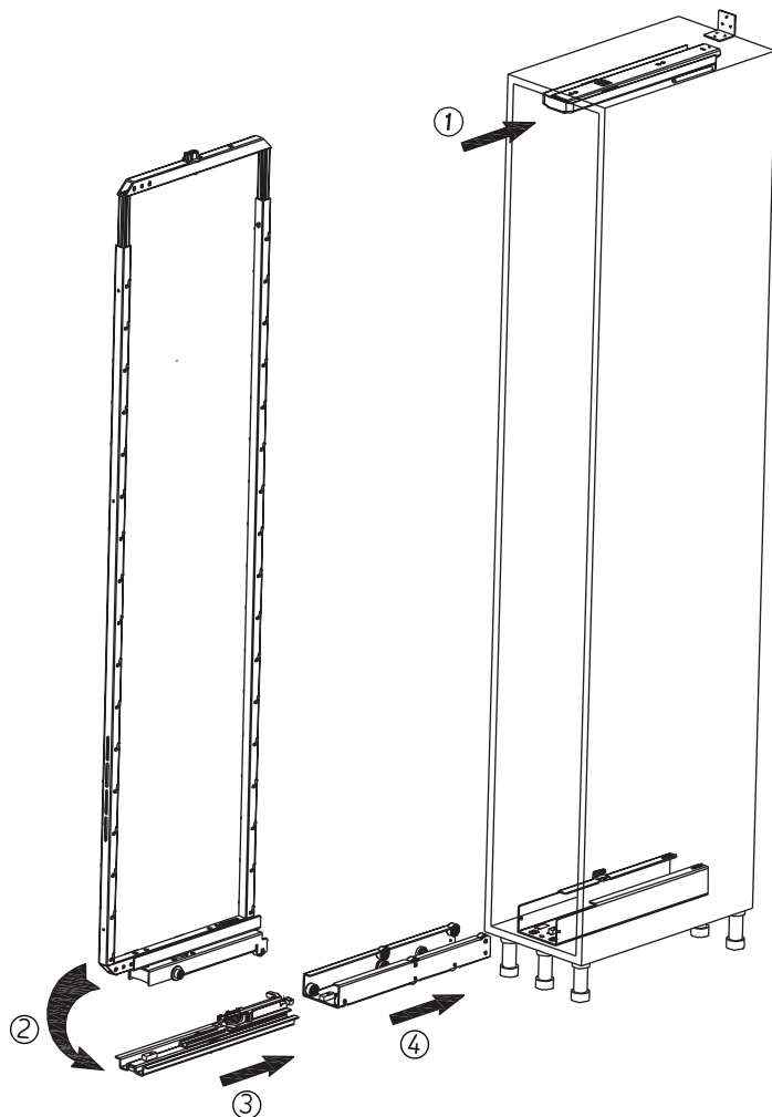
Ensamble del marco extraíble
