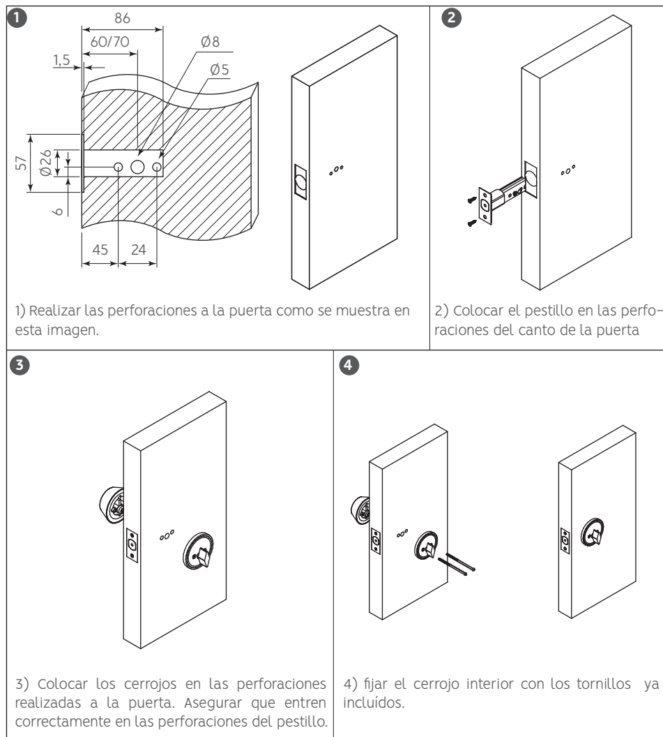
Diagrama de ensamble cerrojo
