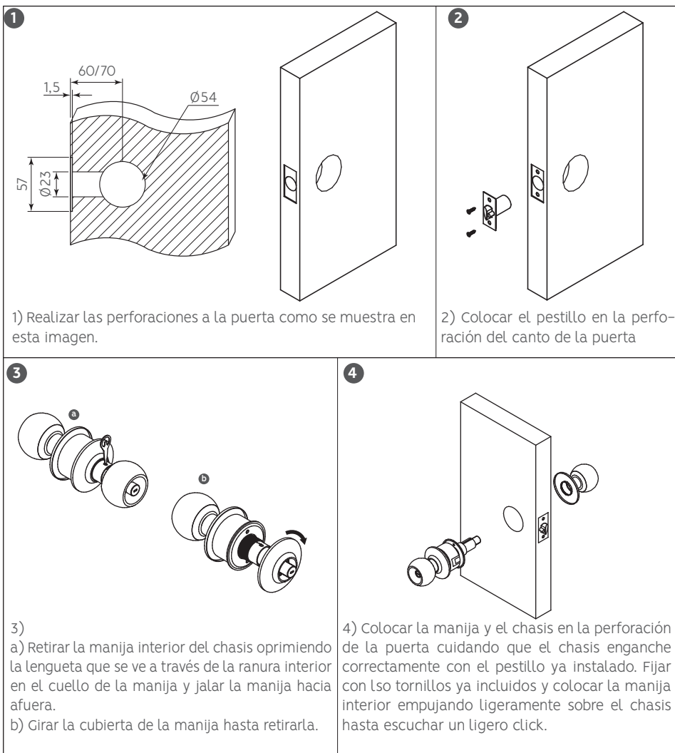
Diagrama de ensamble majina de bola
