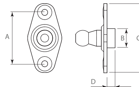
Dimensiones Generales
