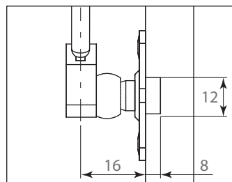
Enganche inferior
