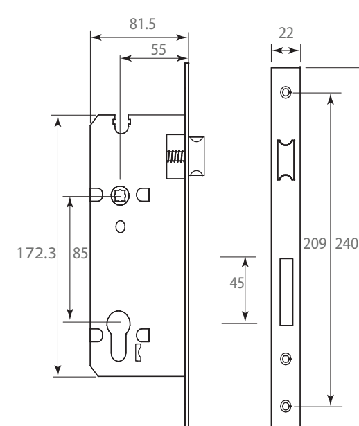
Mecanismo 55x85
