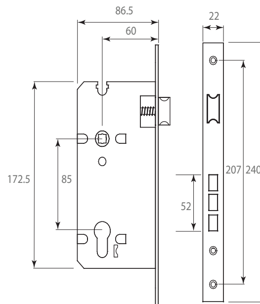
Mecanismo 60x85
