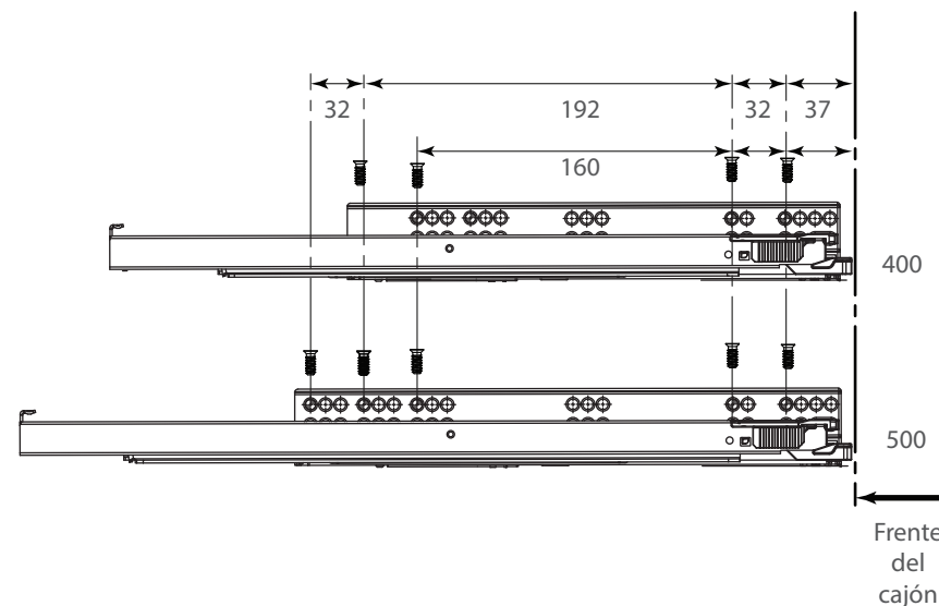
Dimensiones generales
