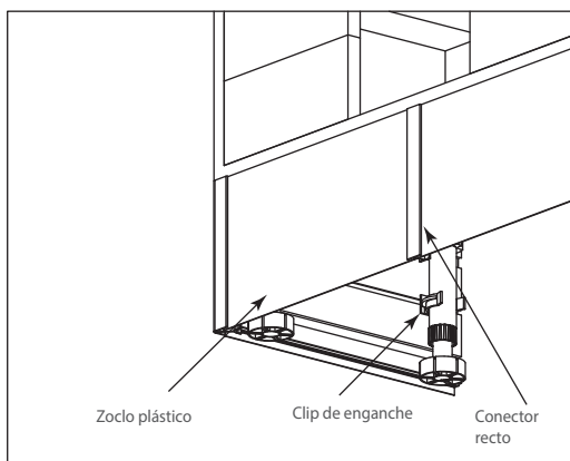
Diagrama de instalación:
