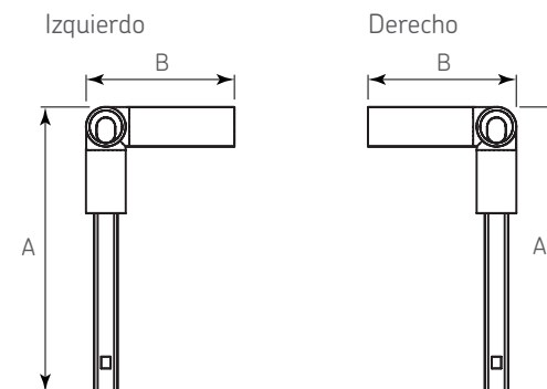
Dimensiones generales
