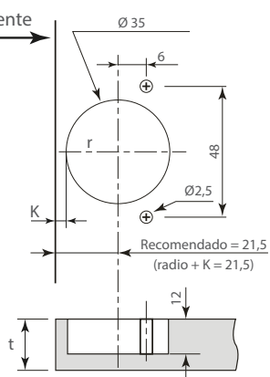
Perforación de la puerta
