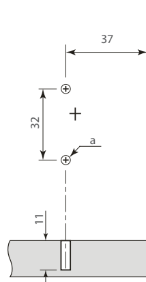
Perforación del gabinete
