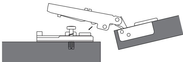
Sistema de montaje:
