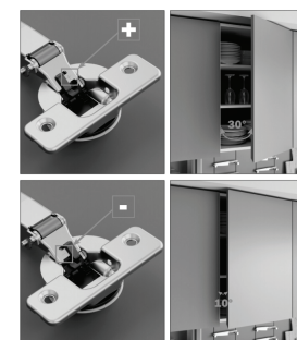
Regulación de la velocidad del cierre suave
