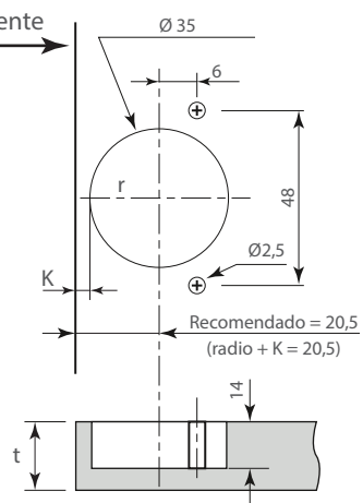
Perforación de la puerta (puerta)
