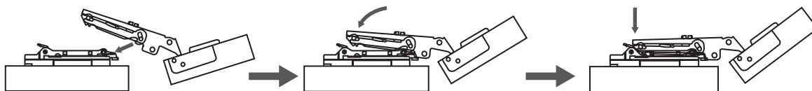
Ensamble de la bisagra en la base
